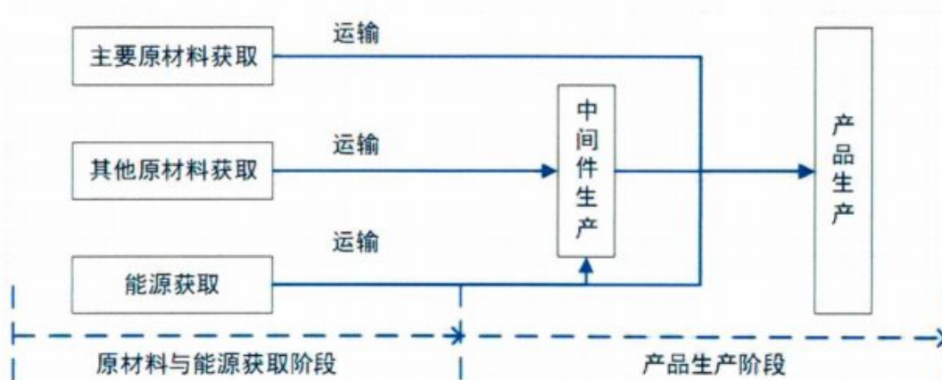
图 1 1 台 SLon-2500 H (1.0T)立环脉动高梯度磁选机碳足迹评价系统边界图
