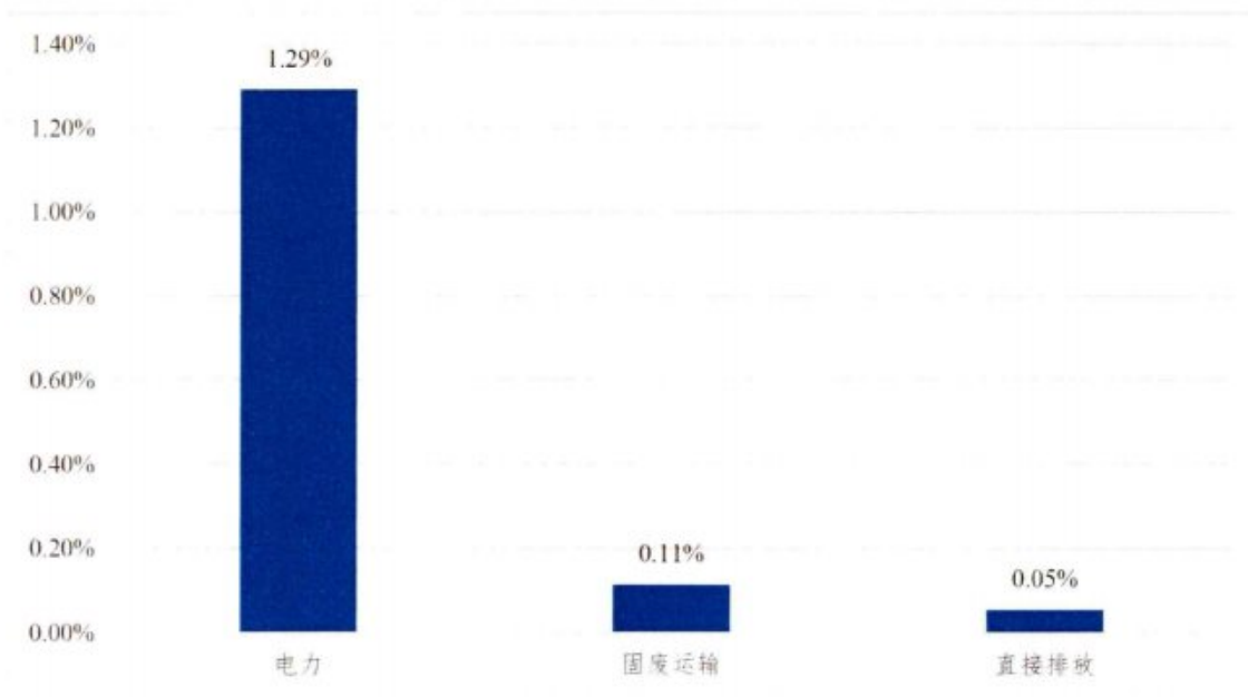
图5 1台 SLon-2500 H (1.0T)立环脉动高梯度磁选机产品生产阶段排放量占比
