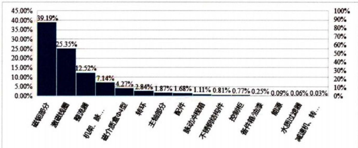
图 2 1 台 SLon-2500 H (1.0T)立环脉动高梯度磁选机产品碳足迹各过程排放量占比
