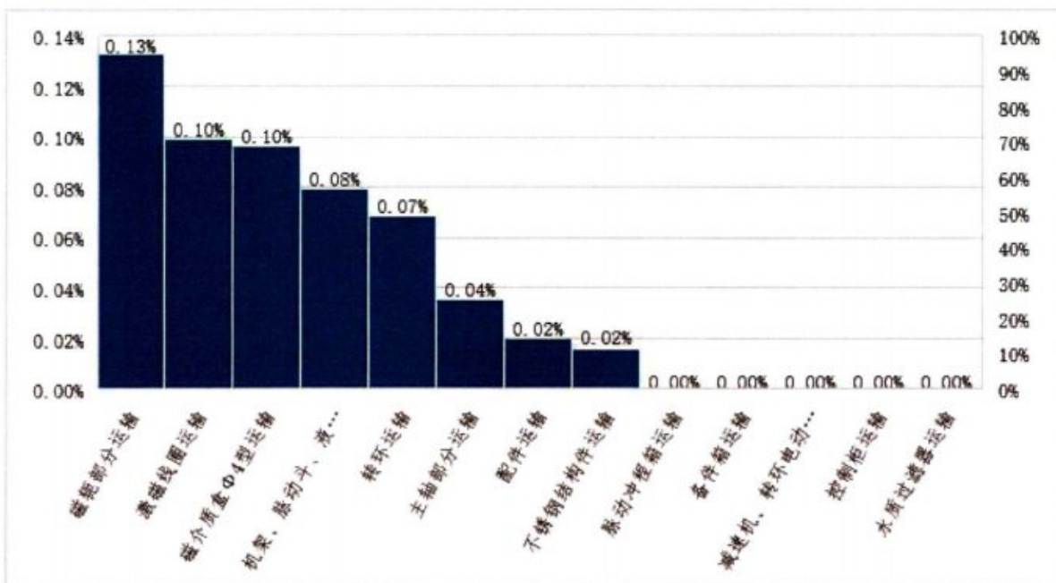
图4 1台 SLon-2500 H (1.0T)立环脉动高梯度磁选机产品原材料运输阶段排放量占比
